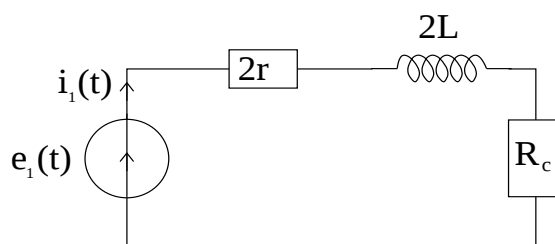
Figure 8 : Schéma équivalent du circuit des bobines ( B_1, B'_1 ).
