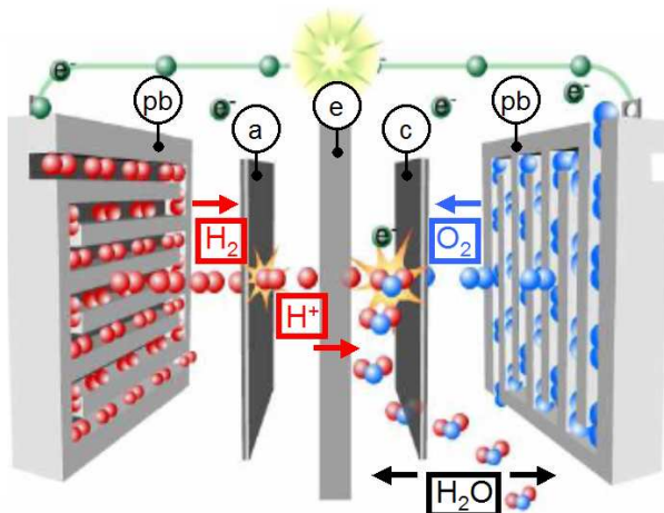
Fig. 1.1 – Principe de la PEMFC, avec : pb : plaque bipolaire, a : anode, e : membrane électrolyte (Nafion), c : cathode
