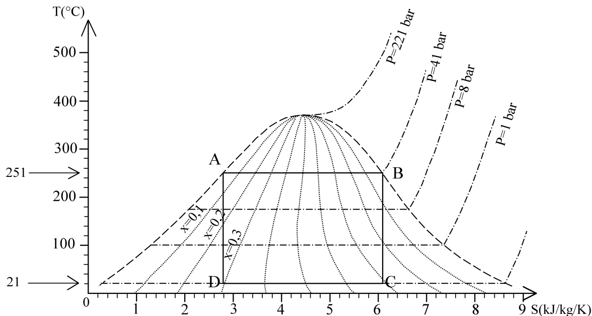
Figure 5 – Cycle de Carnot dans un diagramme entropique de l'eau
