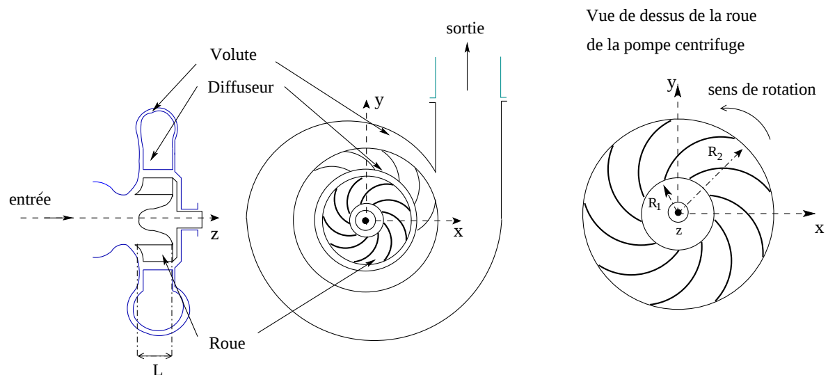
Figure 13 : Représentation schématique d'une pompe centrifuge
