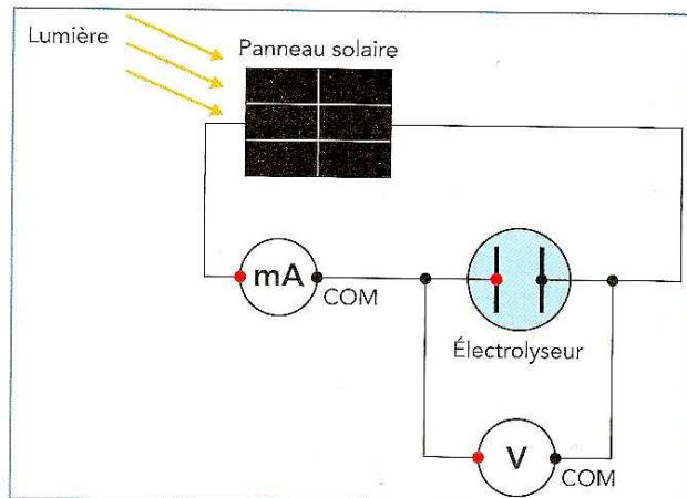
Doc. 5 Production du dihydrogène et du dioxygène.
