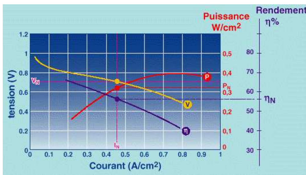
Fig. 6 – Caractéristiques électriques d'une cellule PEMFC
