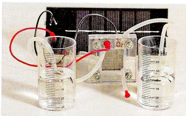
Doc. 4 Cellule constituant la pile à combustible.
