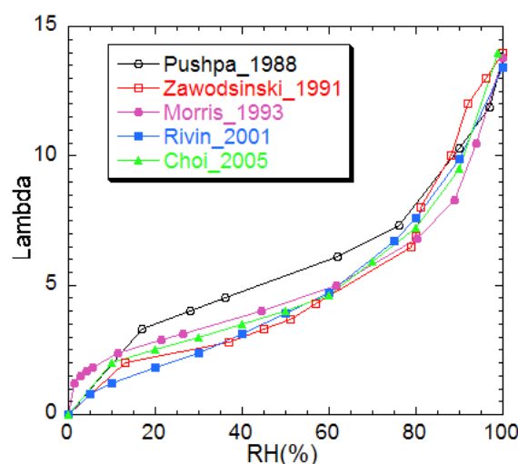
Fig. 1.13 – Isothermes de sorption d'un Nafion 1100 \text{g.eq}^{-1} à 25 °C
