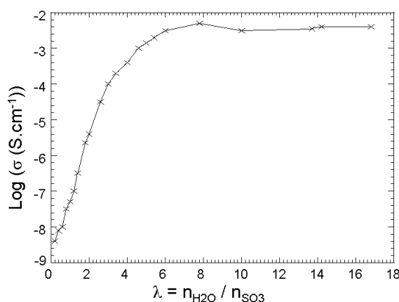
Fig. 1.15 – Conductivité du Nafion 117 en fonction de \lambda à 25 °C
