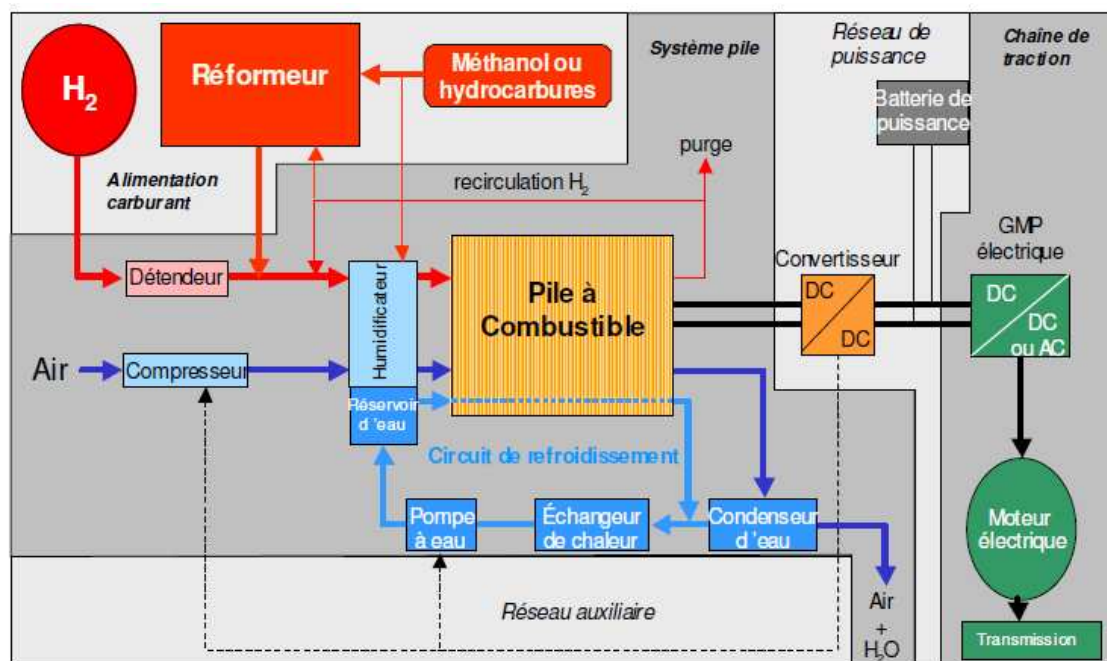
Figure 4 - Schéma général d'un véhicule à pile à combustible - Source Renault – PSA, 1998
