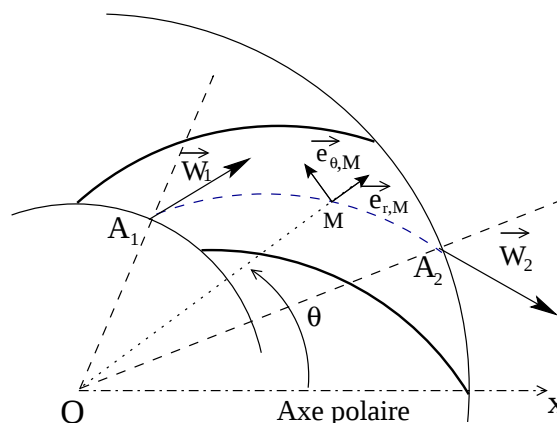
Figure 15 : Trajectoire d'une particule de fluide dans le référentiel lié à la roue
