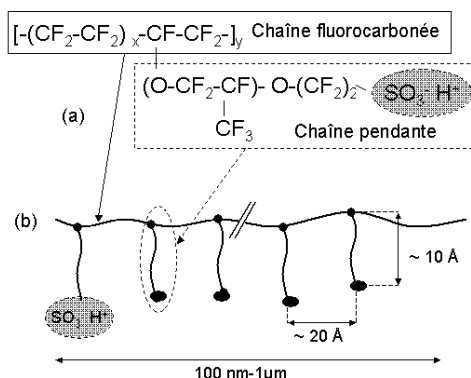
Fig. 1.2 – (a) Formule chimique du Nafion : 5 \leq x \leq 14 et 100 \leq y \leq 1000 et (b) Schéma des chaînes pendantes distribuées sur le squelette perfluoré
